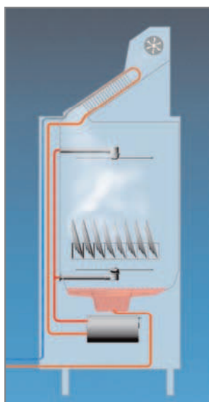
Schématické znázornění procesu zpětného získávání tepla GS 640 Energy (Možné jen při připojení studené vody)
