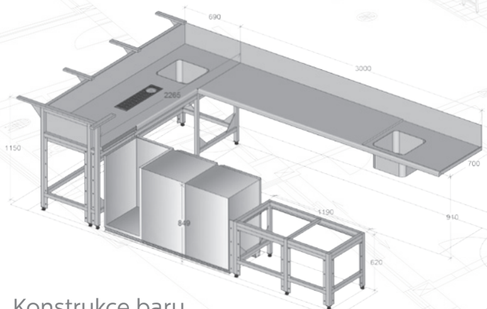
Konstrukce baru kavárny v Brně
